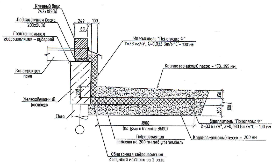
Узел утепления цоколя
